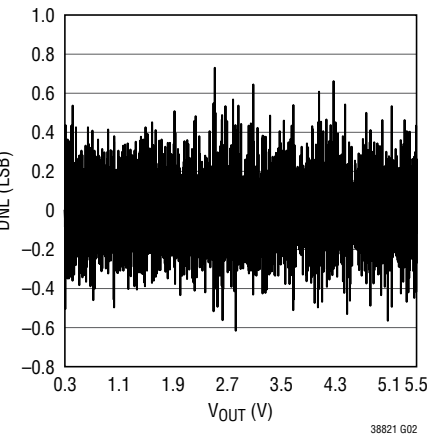
VOUT_COMMAND DNL
