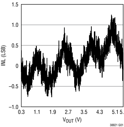
VOUT_COMMAND INL
