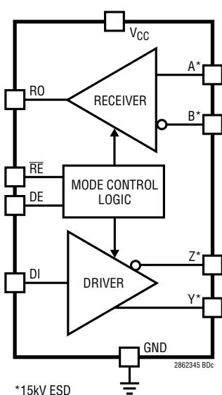
LTC2864
