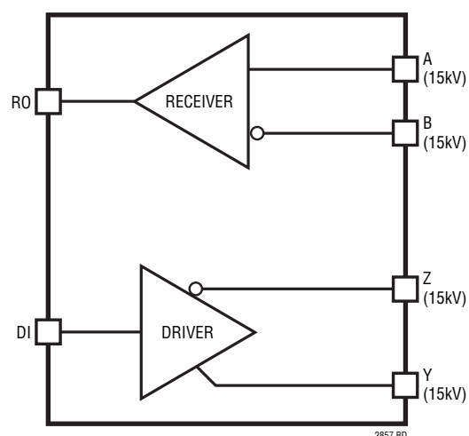
LTC2857-1, LTC2857-2
