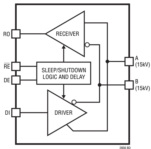
LTC2856-1, LTC2856-2
