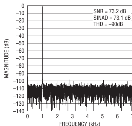
1kHz Sine Wave 8192 Point FFT Plot
