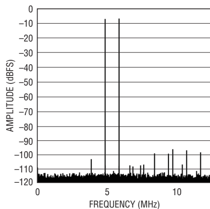
LTC2182: 64k Point 2-Tone FFT, f_{IN} = 69\text{MHz} , 70\text{MHz} , -7\text{dBFS} , 25\text{Mpsps}
