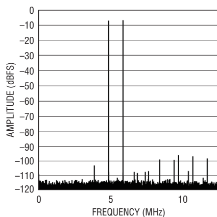
LTC2181: 64k Point 2-Tone FFT, f_{IN} = 69\text{MHz} , 70\text{MHz} , -7\text{dBFS} , 25\text{Mpsps}
