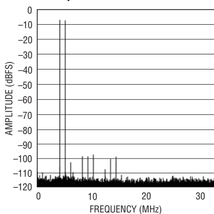
LTC2162: 64k Point 2-Tone FFT, f_{IN} = 69\text{MHz} , 70\text{MHz} , -7\text{dBFS} , 65\text{Mpsps}
