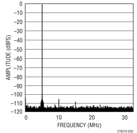
LTC2162: 64k Point FFT, f_{IN} = 5\text{MHz} , -1\text{dBFS} , 65\text{Mpsps}
