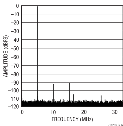
LTC2162: 64k Point FFT, f_{IN} = 70\text{MHz} , -1\text{dBFS} , 65\text{Mpsps}
