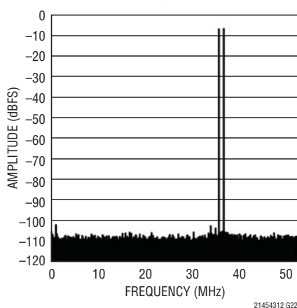
LTC2144-12: 64k Point 2-Tone FFT, f_{IN} = 69\text{MHz} , 70\text{MHz} , -7\text{dBFS} , 105\text{Mps}
