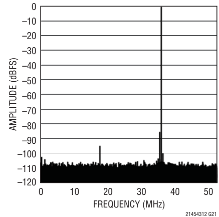
LTC2144-12: 64k Point FFT, f_{IN} = 140\text{MHz} , -1\text{dBFS} , 105\text{Mps}
