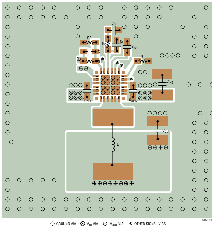
(b) LT8643S
